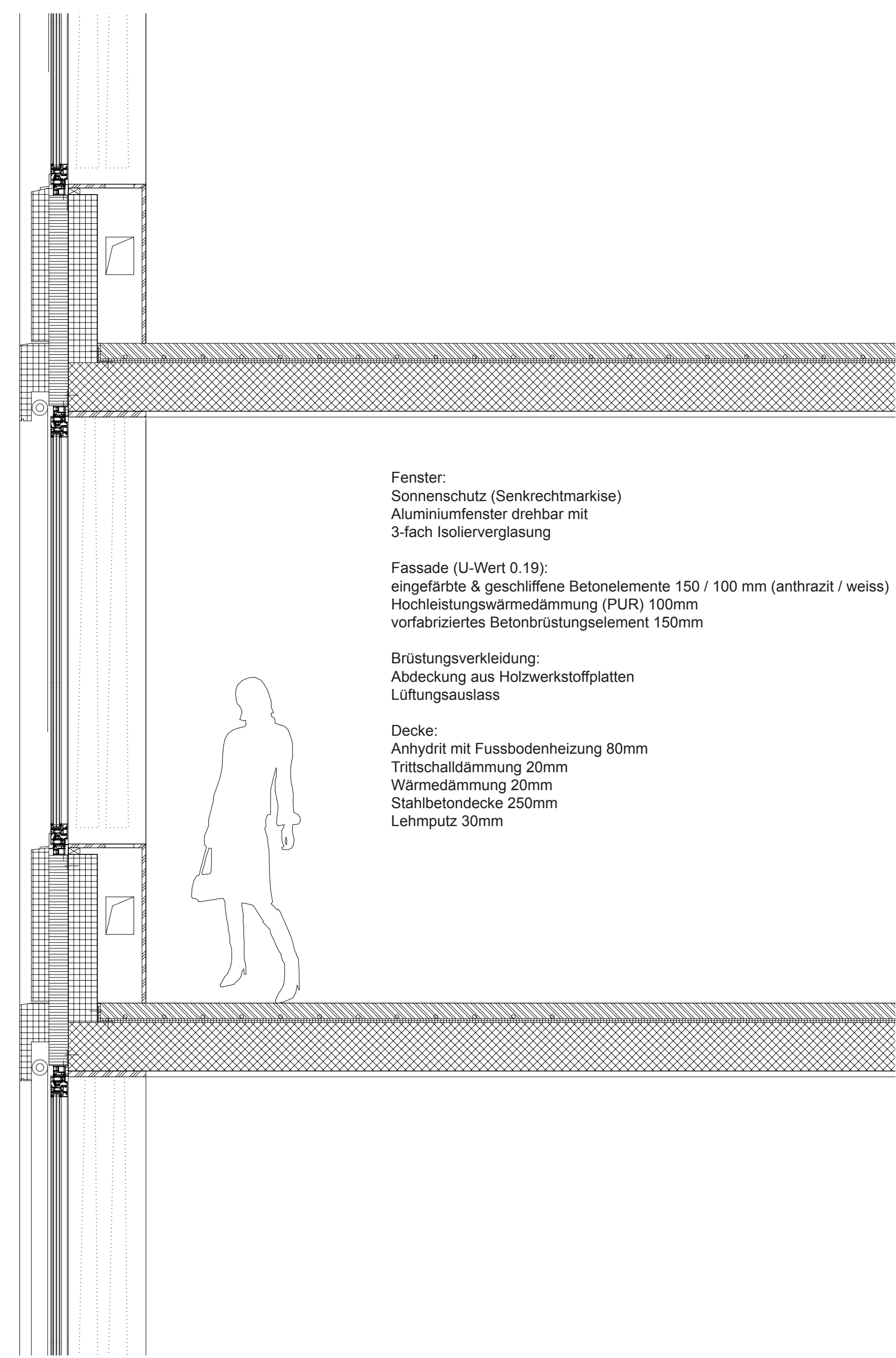
Fassadenschnitt Wohnen 1:20
