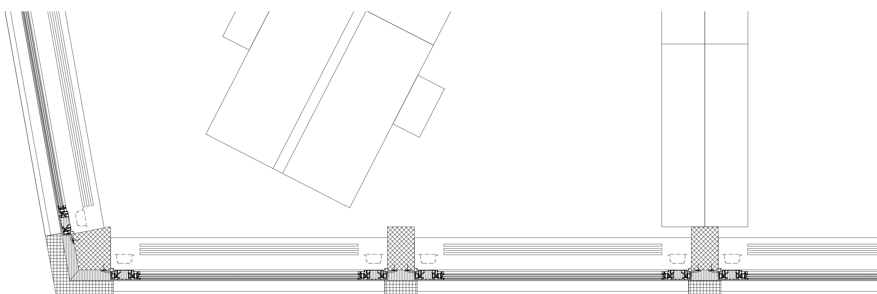
Grundriss Büro 1:20
