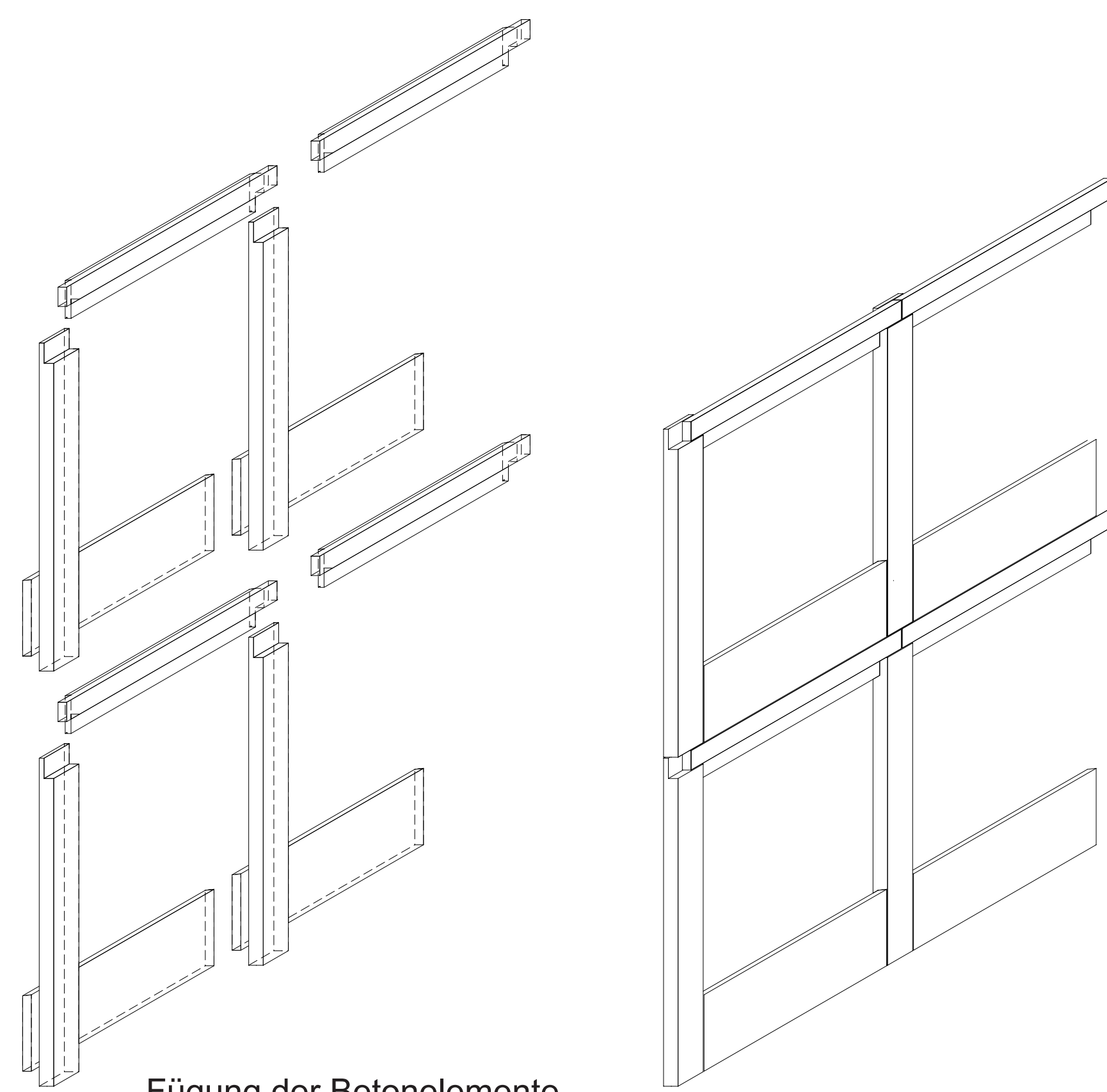
Fügung der Betonelemente
