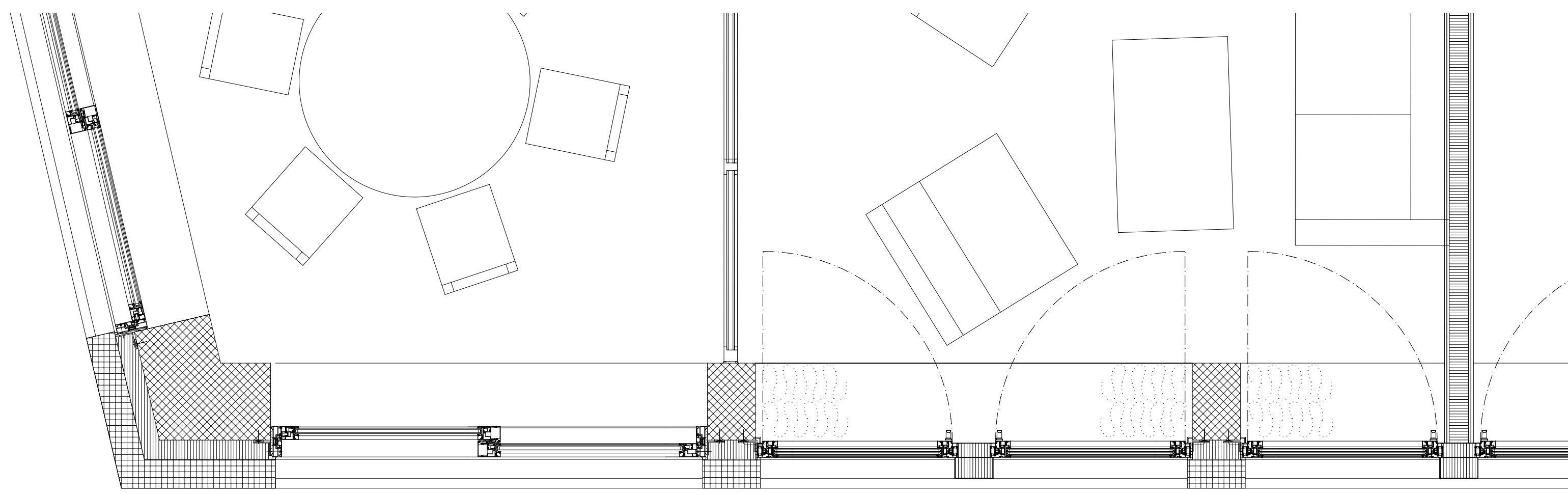
Grundriss Wohnen 1:20
