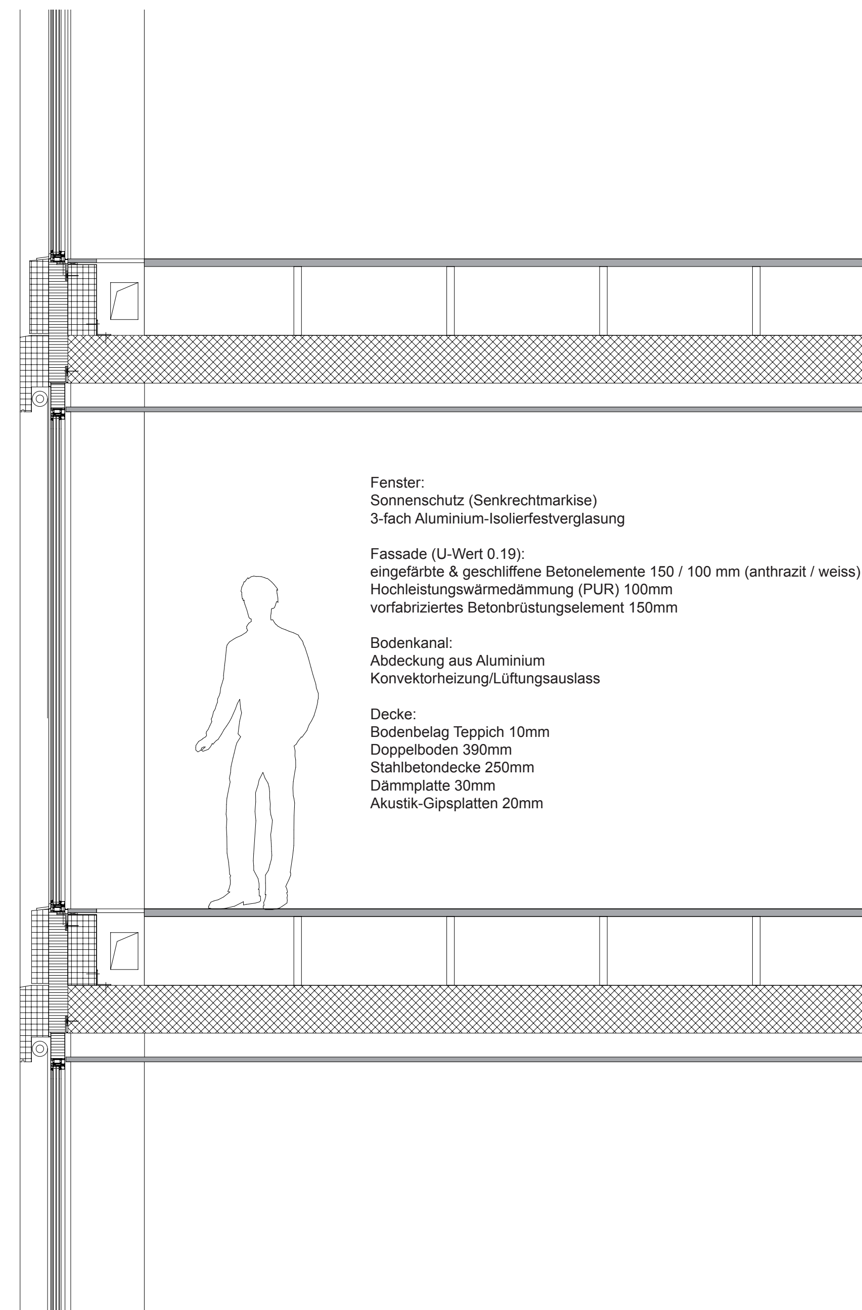
Fassadenschnitt Büro 1:20
