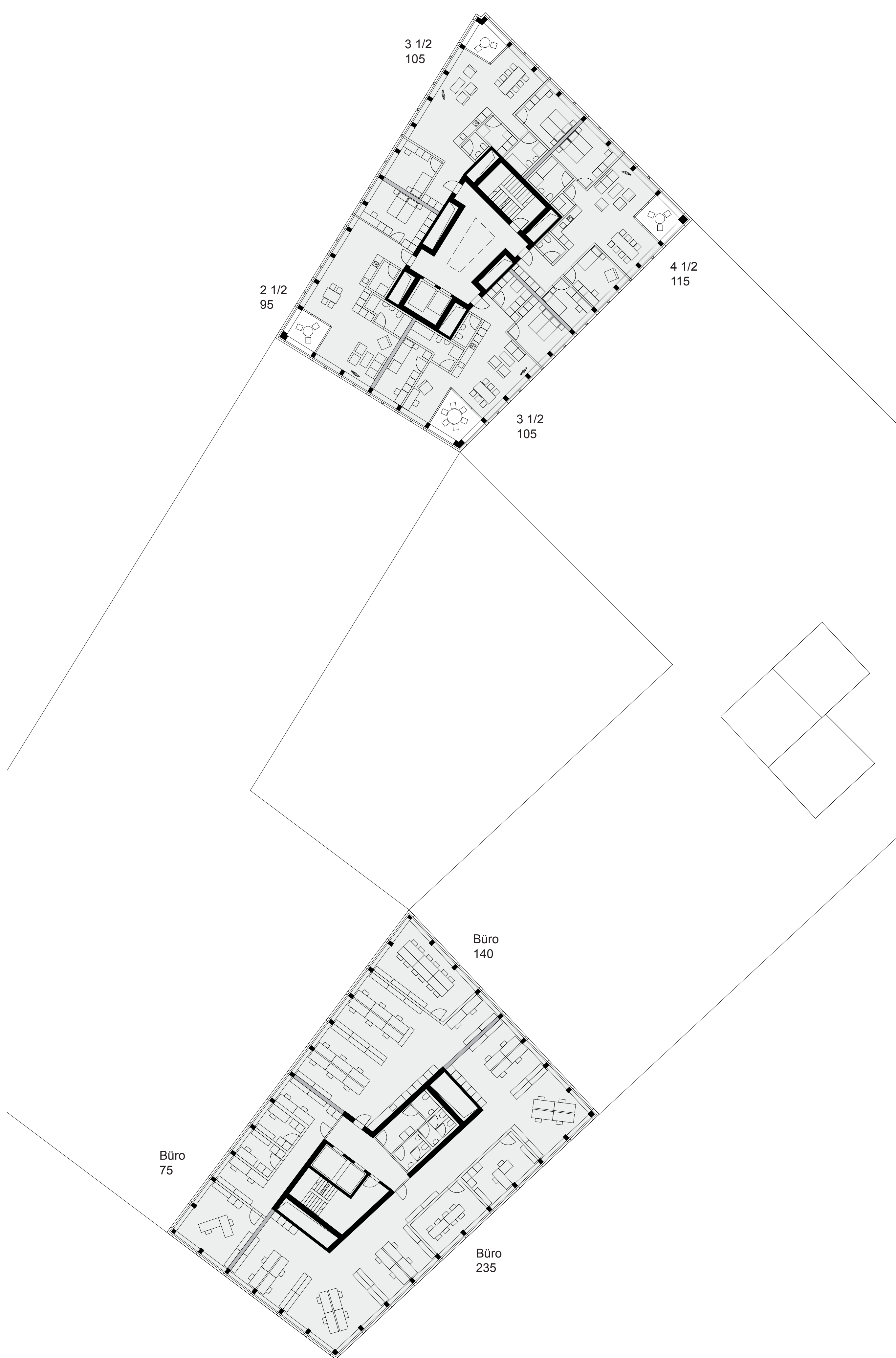
Grundriss Regelgeschoss 1 1:200
