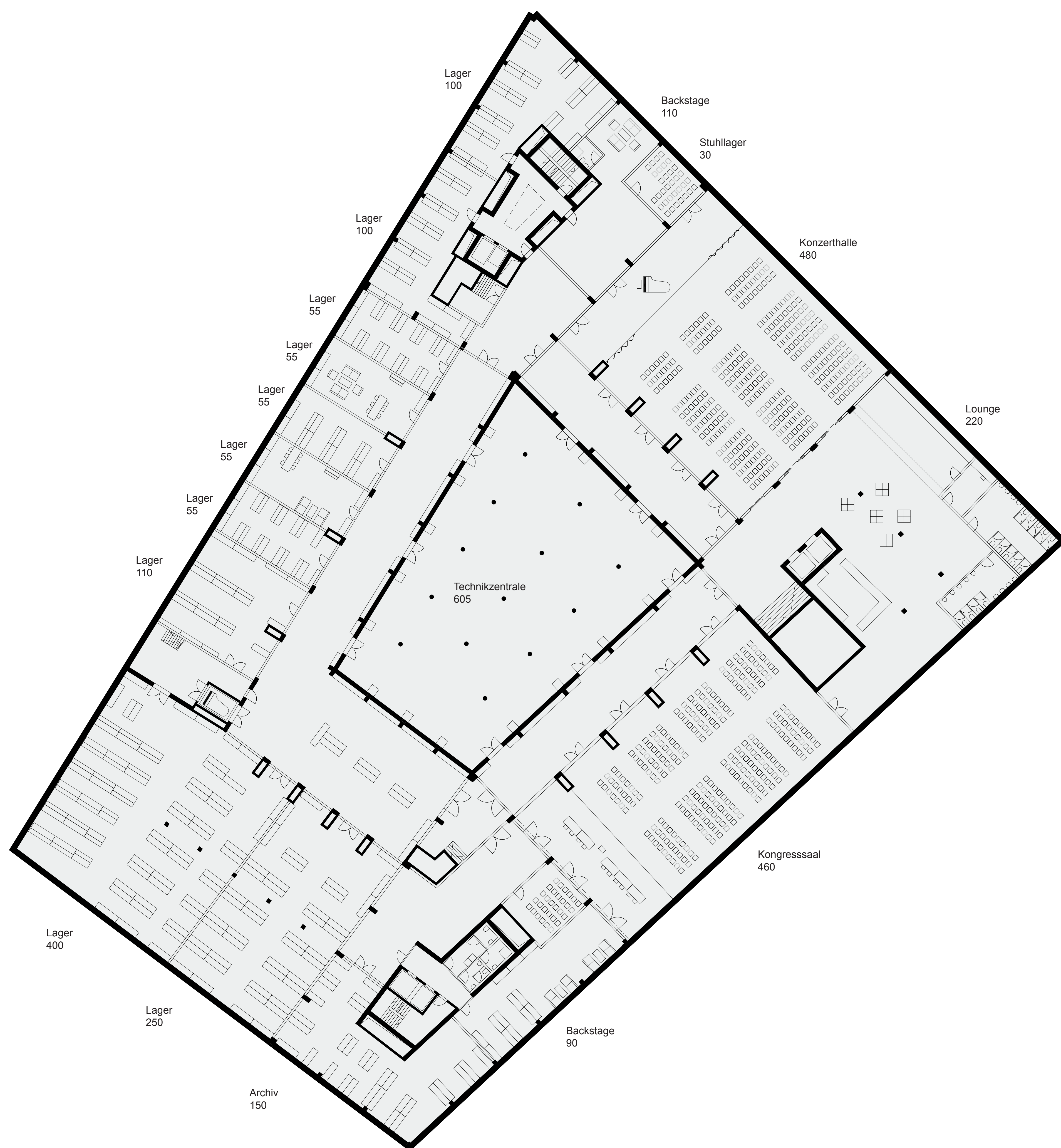
Grundriss UG2 1:200
